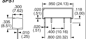
Fig. 2 SPST
