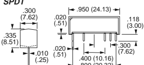
SPDT
