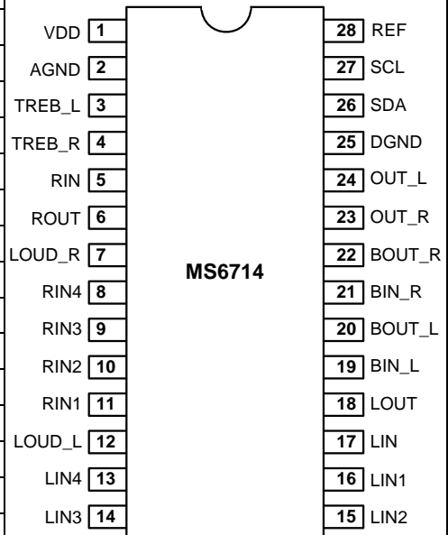
SOP28 / SSOP28
